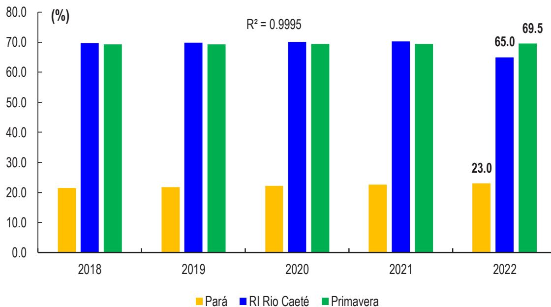
Gráfico 25: Percentual de área desmatada, Pará, Região de Integração Rio Caeté e Primavera, 2018 a 2022.
