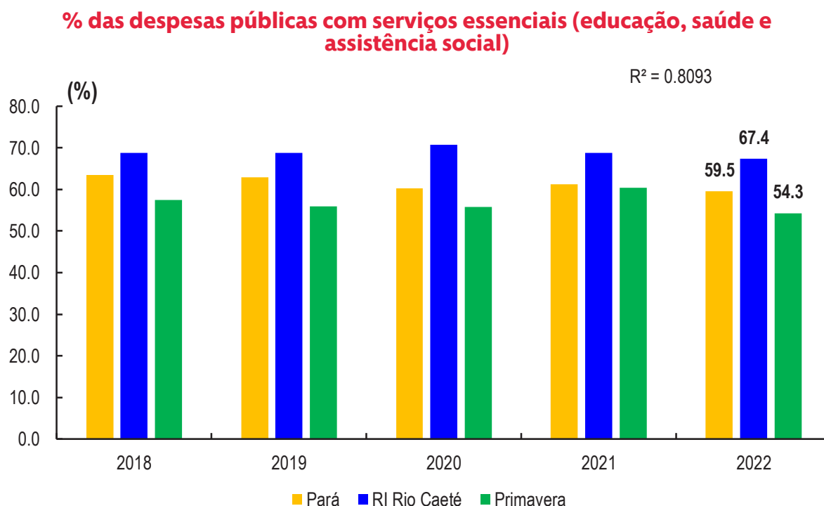
Gráfico 02: Percentual do total das despesas públicas com serviços essenciais (educação, saúde e assistência social), Pará, Região de Integração Rio Caeté e Primavera, 2018 a 2022.
