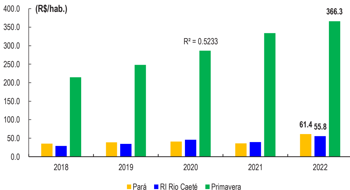
Gráfico 19: Despesa pública municipal per capita com cultura e gestão ambiental, Pará, Região de Integração Rio Caeté e Primavera, 2018 a 2022.
