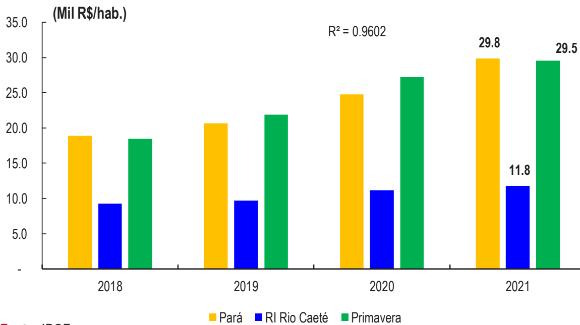
Gráfico 14: PIB per capita, Pará, Região de Integração Rio Caeté e Primavera, 2018 a 2021.
