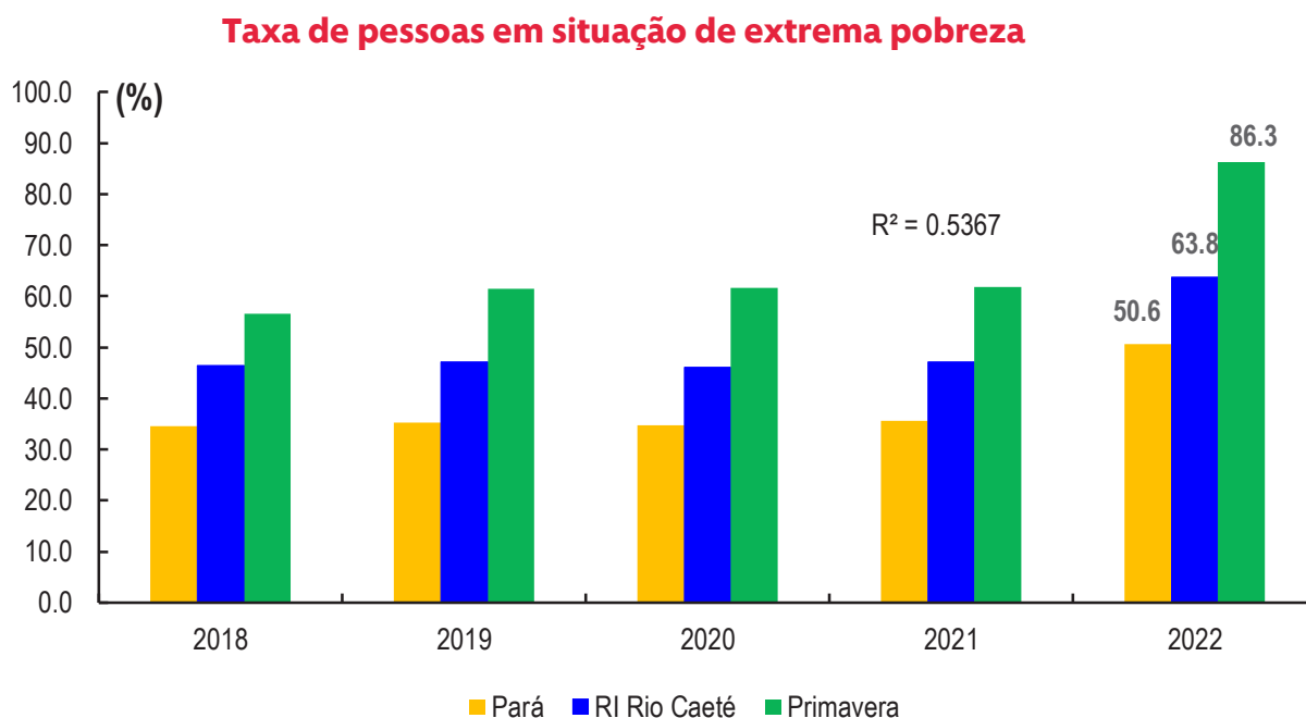
Gráfico 01: Taxa de pessoas em situação de extrema pobreza, Pará, Região de Integração Rio Caeté e Primavera, 2018 a 2022.
