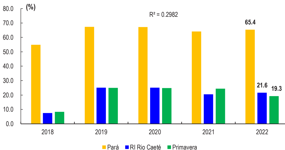
Gráfico 26: Percentual de área de floresta, Pará, Região de Integração Rio Caeté e Primavera, 2018 a 2022.
