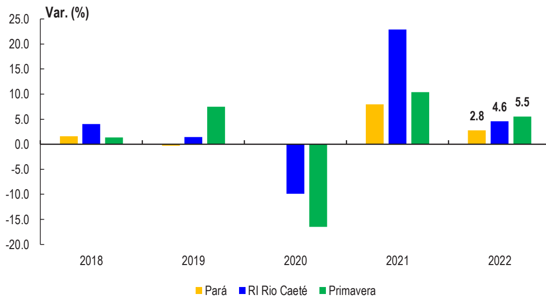
Gráfico 15: Criação de vínculos formais, Pará, Região de Integração Rio Caeté e Primavera, 2018 a 2022.
