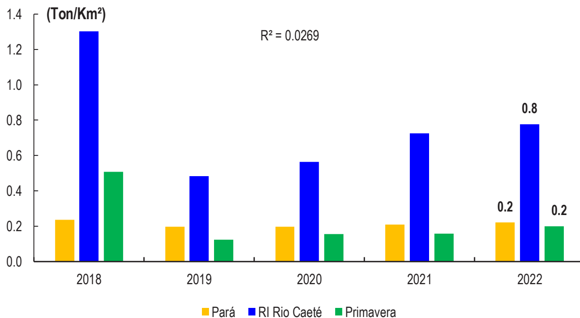
Gráfico 22: Produtividade de produtos florestais não madeireiros, Pará, Região de Integração Rio Caeté e Primavera, 2018 a 2022.
